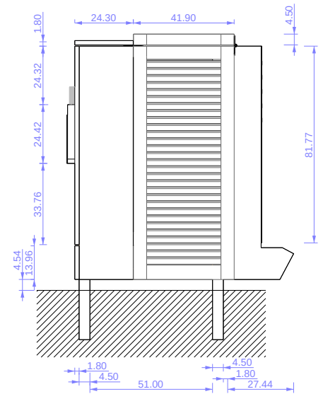
Πλάγια όψη
