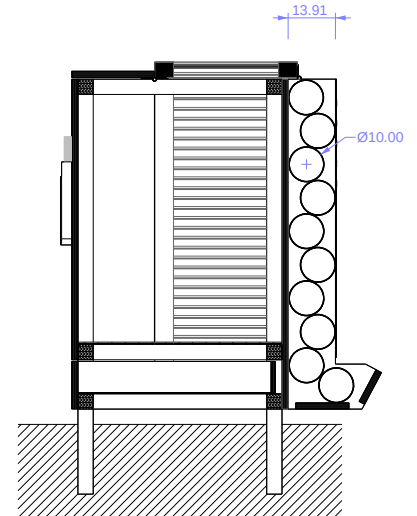
Τομή A/A
